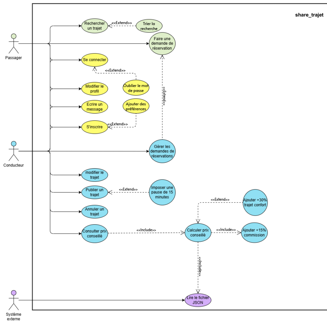
Diagramme de cas d'utilisation qui illustre les interactions principales entre les acteurs et le système
